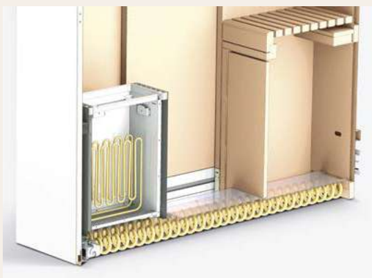
TECHNIQUE INVISIBLE : tous les raccords du poêle VARIUS sont cachés dans le canal multifonctions.
